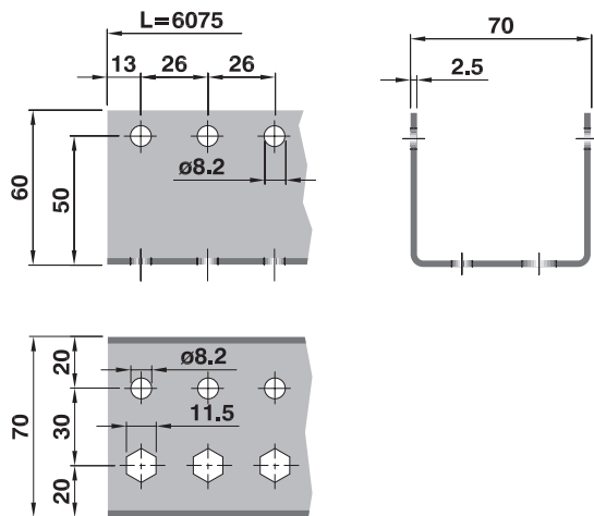
Profilo-Profile PR U50 6075
