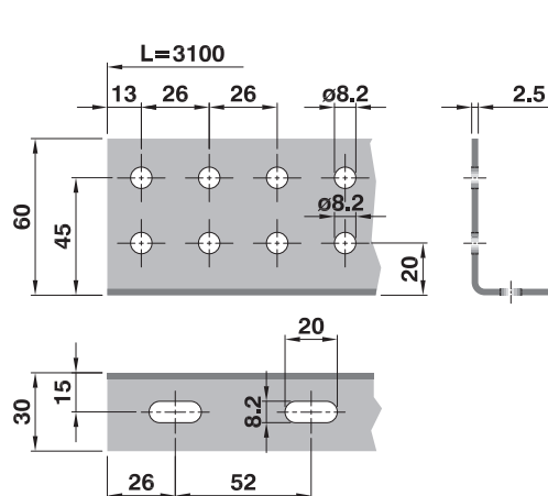
Profilo-Profile PR L60 3100
