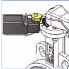
KFC10g Kit interruttori di fine- corsa per segnalazione Aperto/Chiuso (esclusa serie Jg.000/Lg.000) Limit switches kit (exclu- ded series Jg.000/Lg.000) (Jg DN 25-400 Lg DN 25-300)
