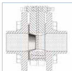
Deflettore conico per Serie 19 Conical deflector for Series 19
