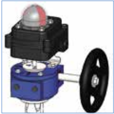
KBOXRM Kit box Micro per riduttore manuale Limit switch box for gear box kit (Jg DN 25-400 Lg DN 25-300)
