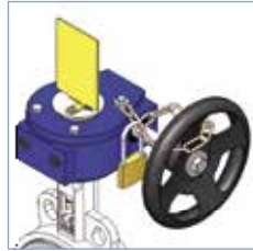
KPOSRM.0250+L Indicatore visivo e lucchettaggio per ridut- tore manuale Position indicator and padlocking for gear box (Jg DN 25-400 Lg DN 25-300)
